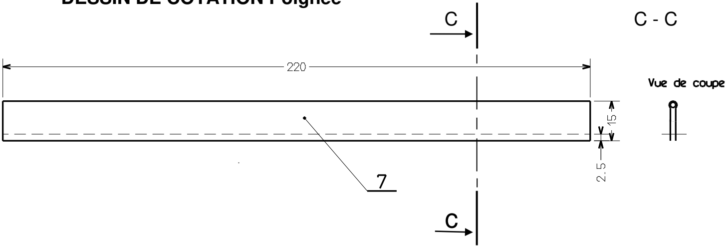
DESSIN DE COTATION Poignée
